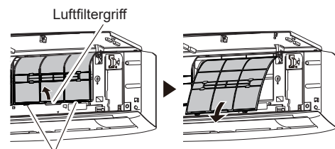
Zapfen (2 Stellen)
