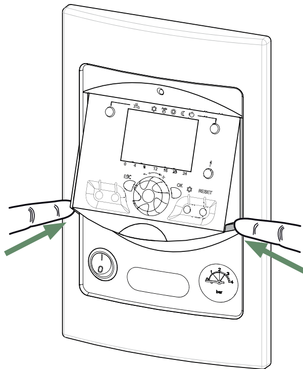
fig. 2 - Fermeture de l'afficheur
