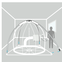
8. 將支條的末端插入位於基底角落處的錨定點。
