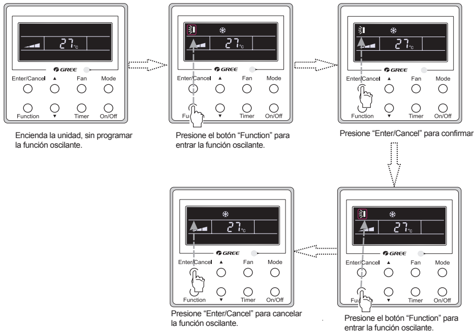
Fig. Programación función oscilante
