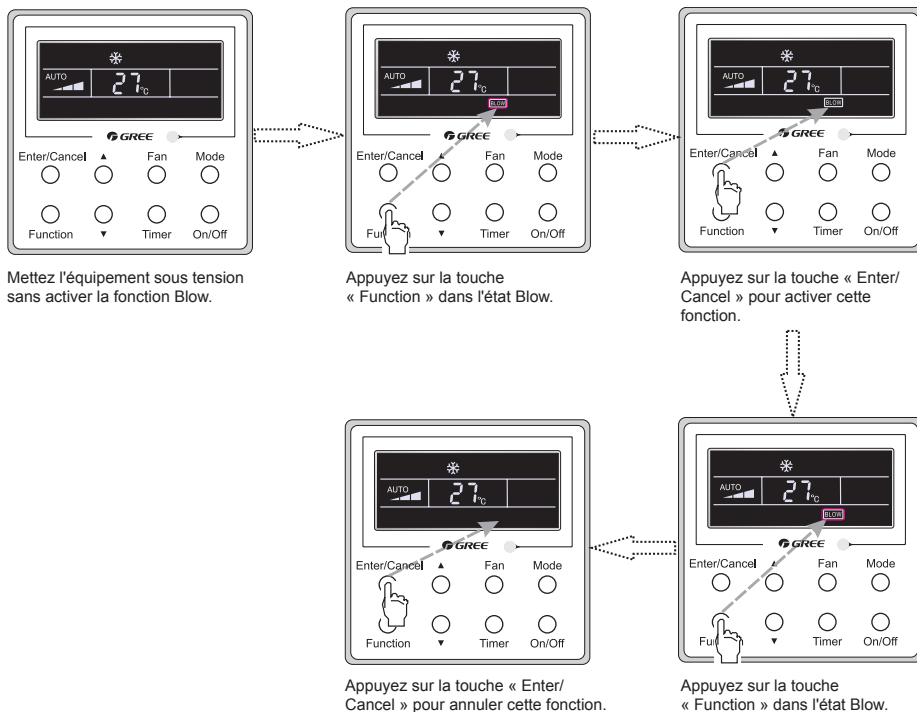
Fig.13 Réglage Blow
