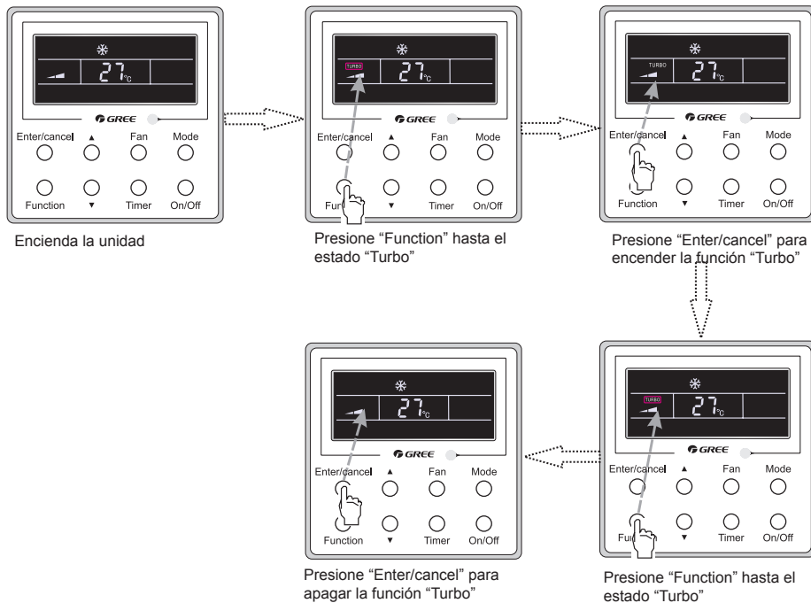
Fig.11 Programación función Turbo
