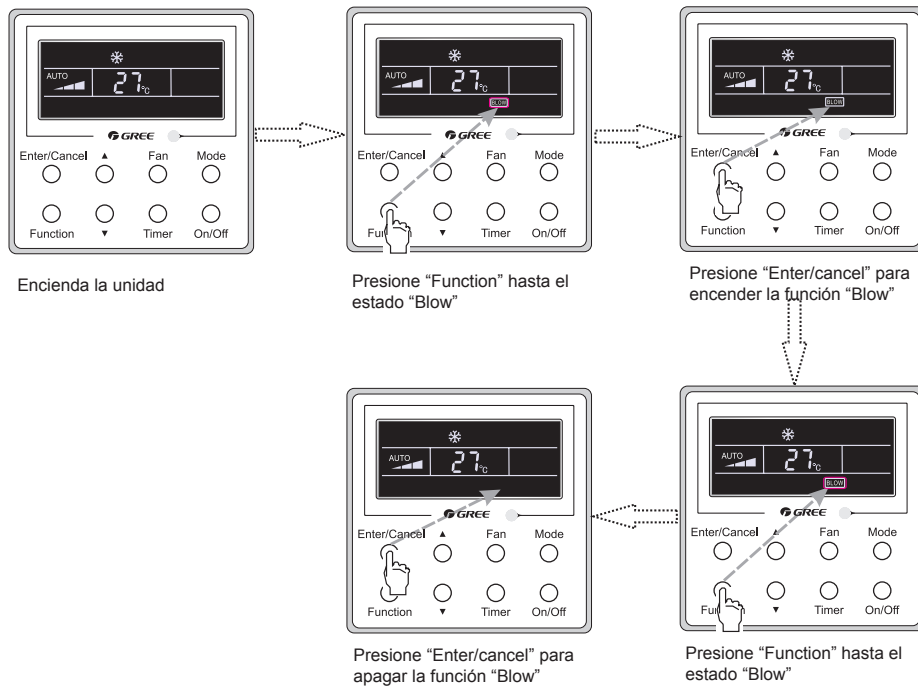
Fig.13 Programación Secado
