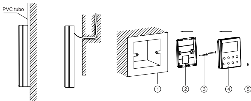
Fig.14 Accesorios para la instalación del termostato
