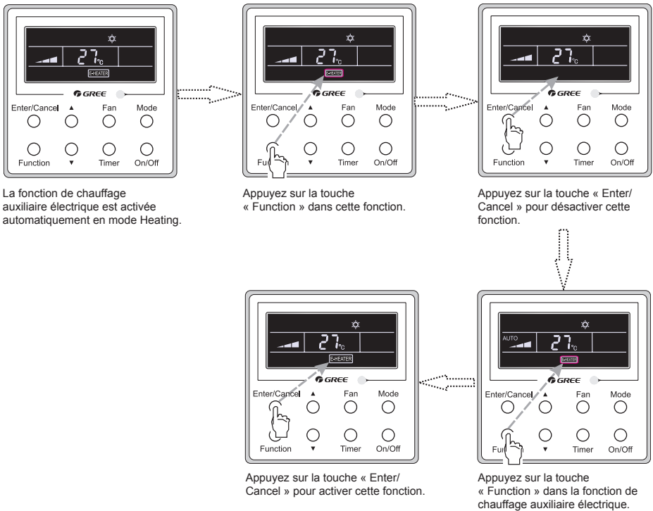
Fig.12 Réglage E-heater
