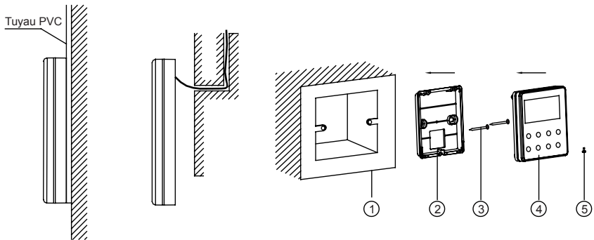
Fig.14 Accessoires d'installation du contrôleur à distance câblé
