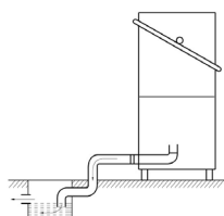
Évacuation libre
