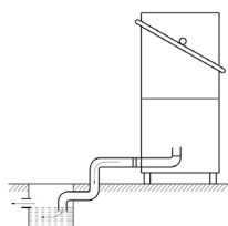
Escoamento livre
