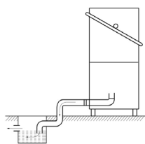
Ελεύθερη αποχέτευση
