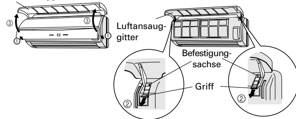
Luftansauggitter
