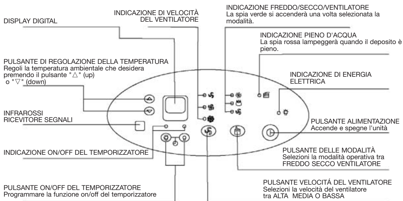
Asse dei comandi
