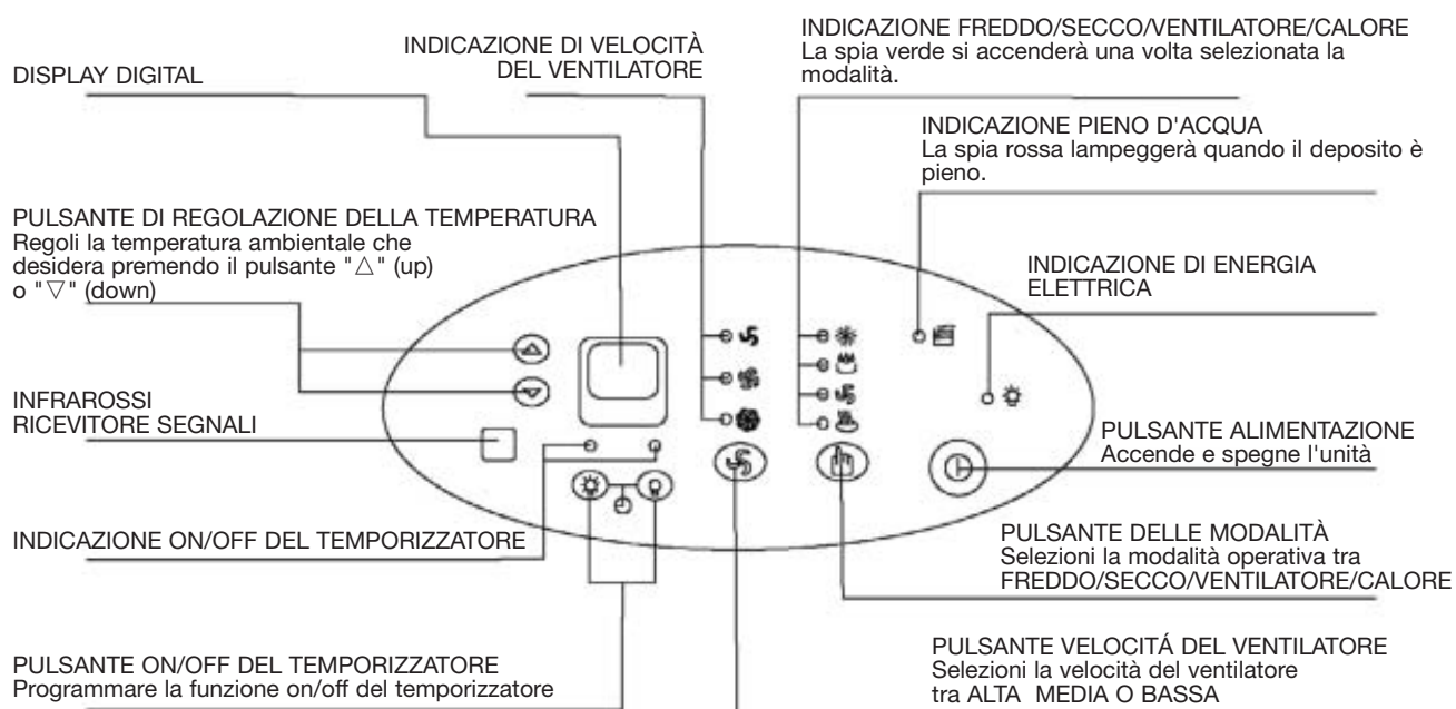
Asse dei comandi
