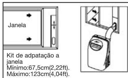
Kit de adaptação a janela Mínimo:67,5cm(2,22ft). Máximo:123cm(4,04ft).
